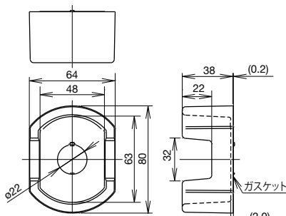
HW9Z-KG1形
