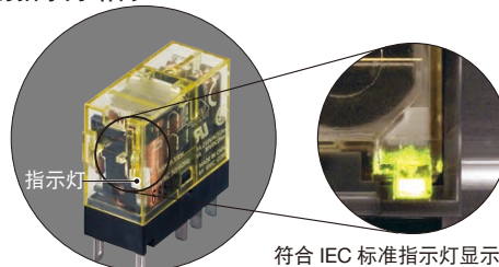
• 独特的指示灯结构
