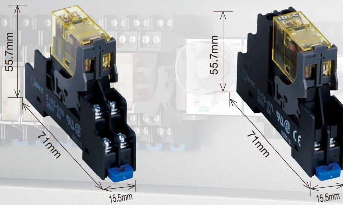
[安装到插座时]
